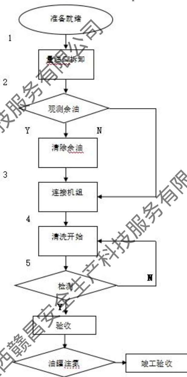
图 2.7-1 清罐流程图
